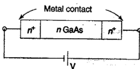
Fig: Gunn Diode
